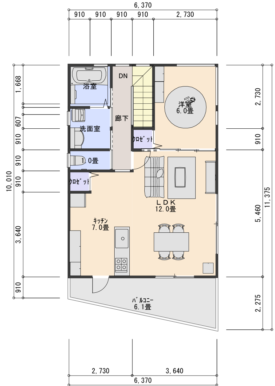
2階 縮尺 1/100
