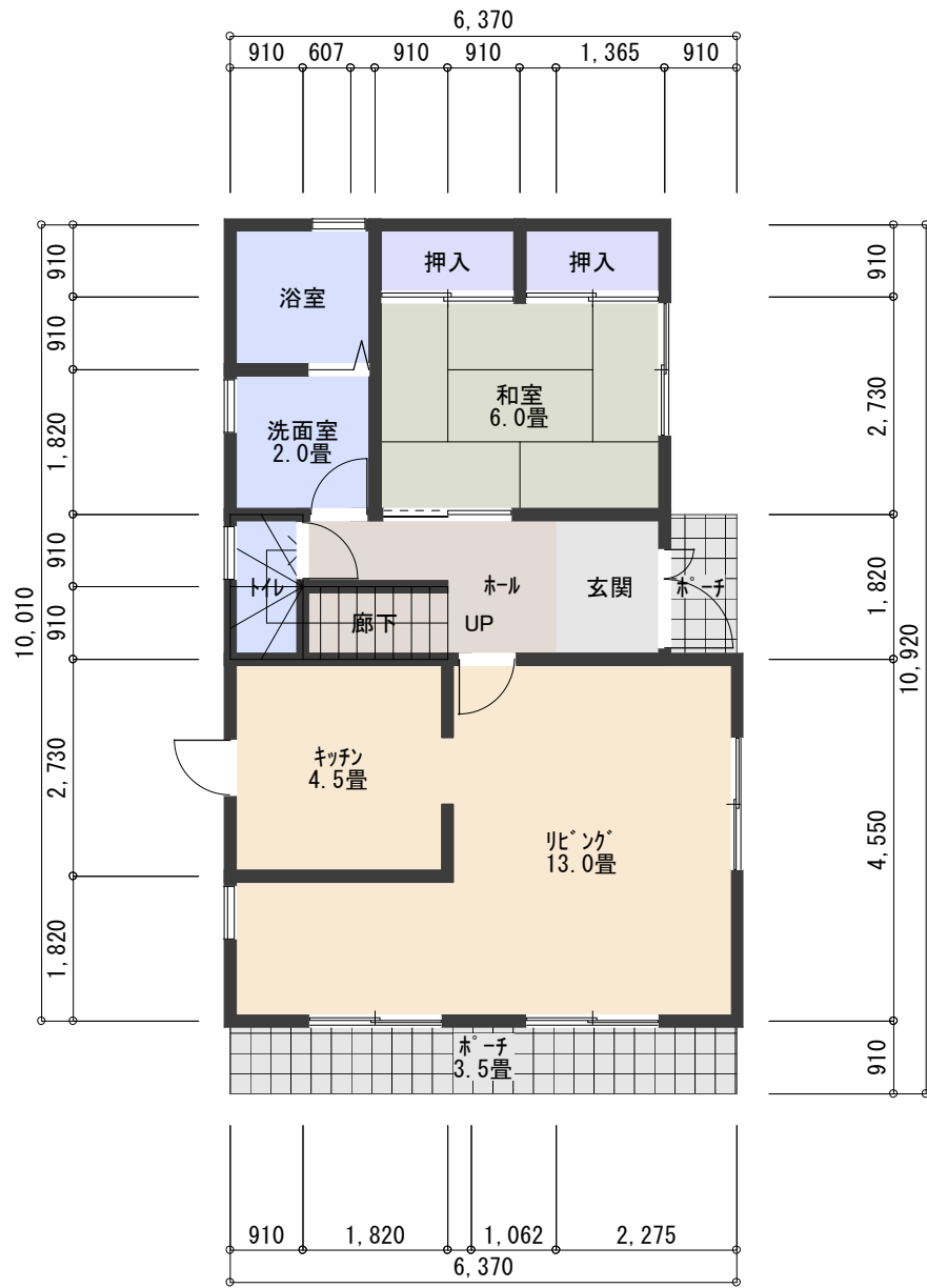
1階 縮尺 1/100
